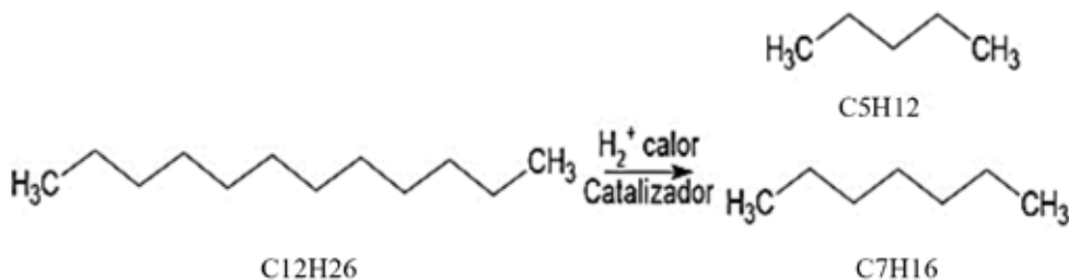
Figura 2.17. Hidro craqueo catalítico
